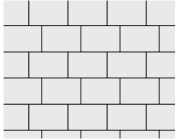
Voorbeeld 2 - Benodigd per m 2 • 30 x 20 cm - ca. 17 stuk
