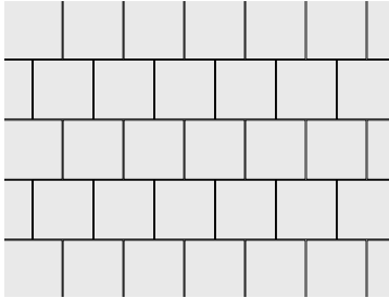
Voorbeeld 1 - Benodigd per m 2 • 20 x 20 cm - ca. 25 stuk
